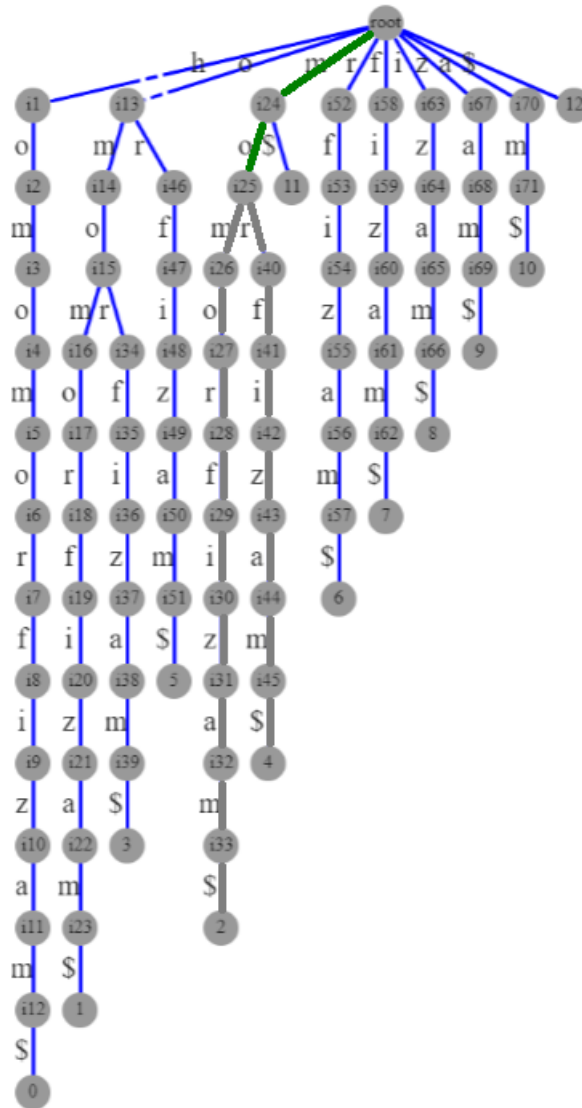
Slika 2.8: Više rešenja poklapanja šablona mo u niski genoma homomorfizam. Poklapanja se nalaze na pozicijama 2 i 4.
