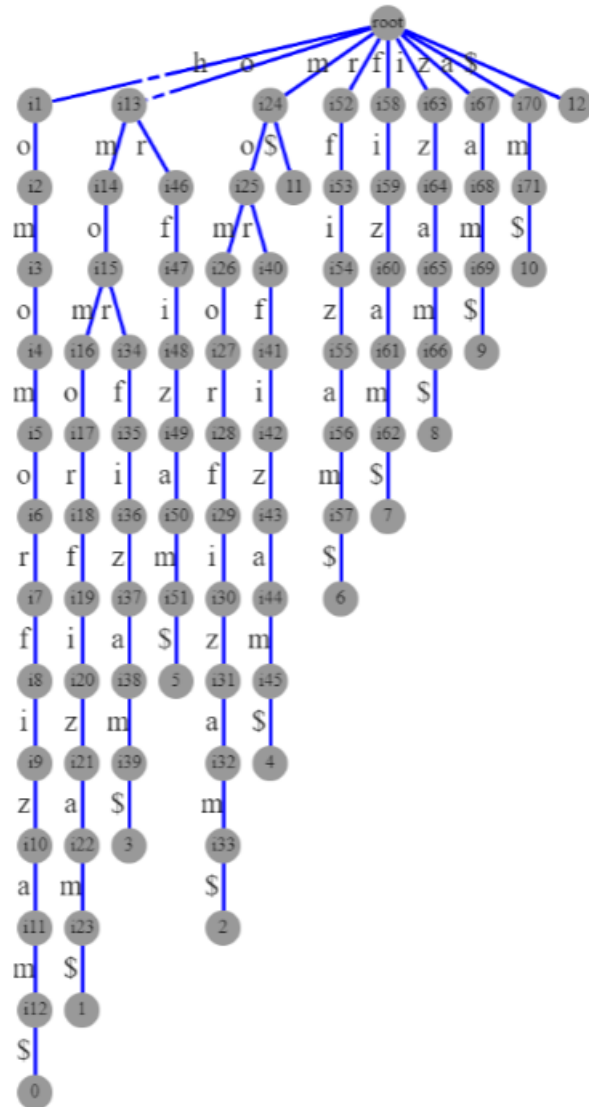
Slika 2.5: Sufiksno stablo za primer genoma homomorfizam
