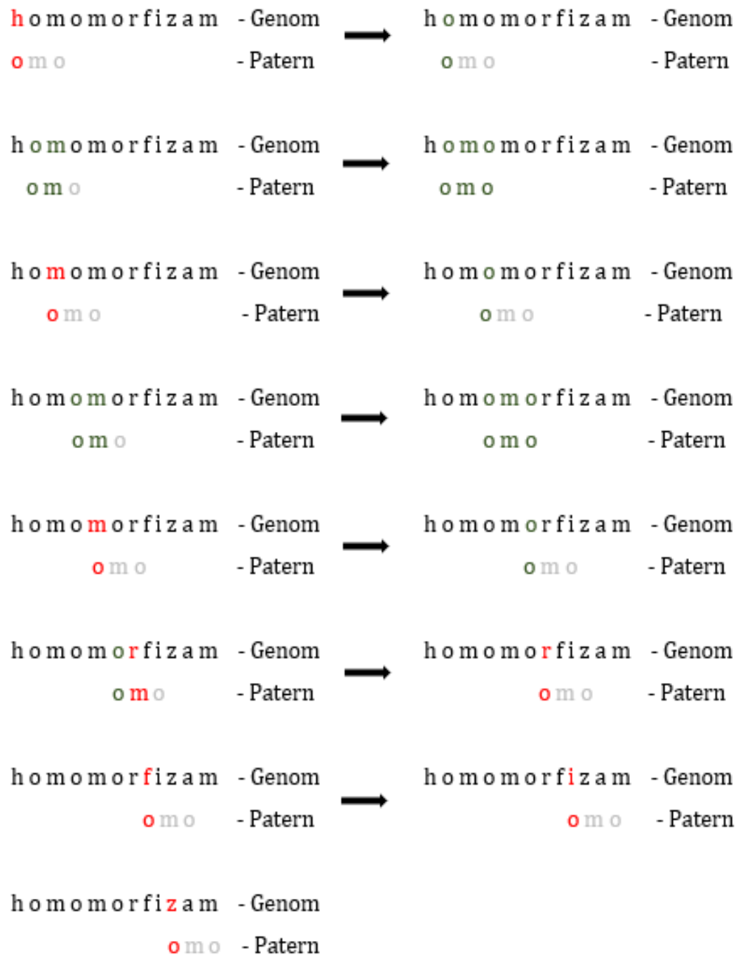
Slika 2.1: Primer korišćenja iterativnog algoritma na primeru genoma homomorfizam i šablona omo
