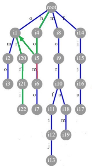
Slika 2.31: Sufiksni link posle čvora o u stablu sa slike 2.30, omogućava nam da možemo da skočimo sa putanje koja počinje sa ho , na putanju koja počinje sa o .
