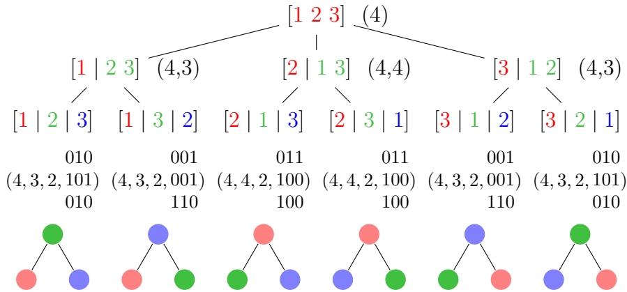
Slika 2.8: Invarijanta stabla.
