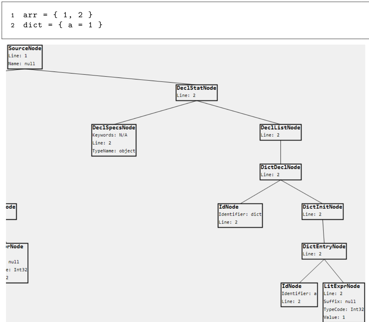
Slika 3.12: Primer deklaracije niza i mape u programskom jeziku Lua i deo odgovarajućeg AST.
