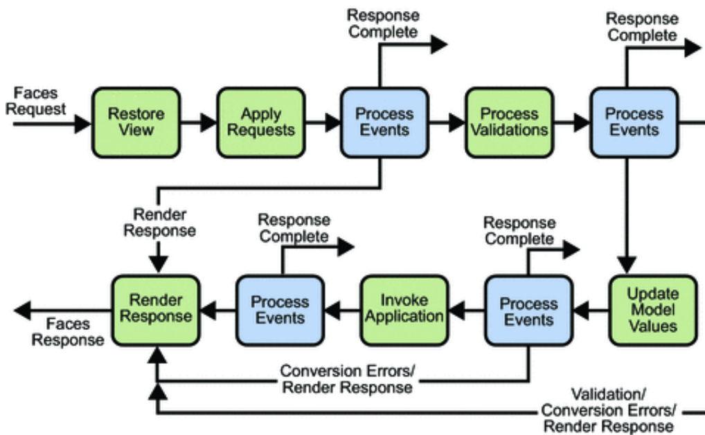
Слика 2: Фазе животног циклуса захтева
