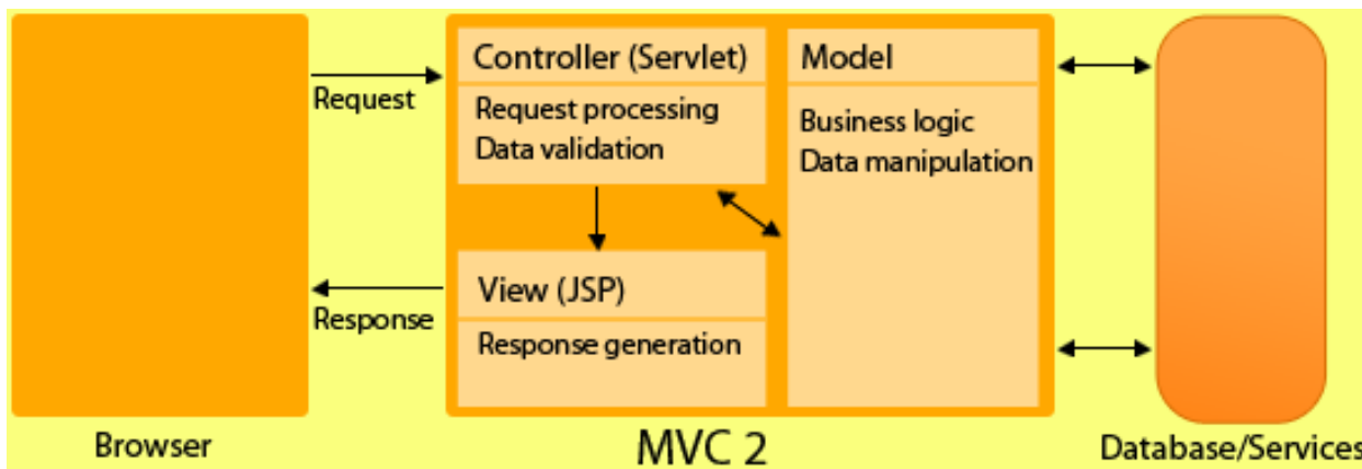
Слика 1: Архитектура MVC2
