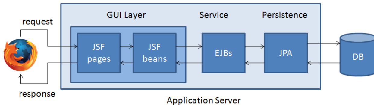
Слика 14: Архитектура система
